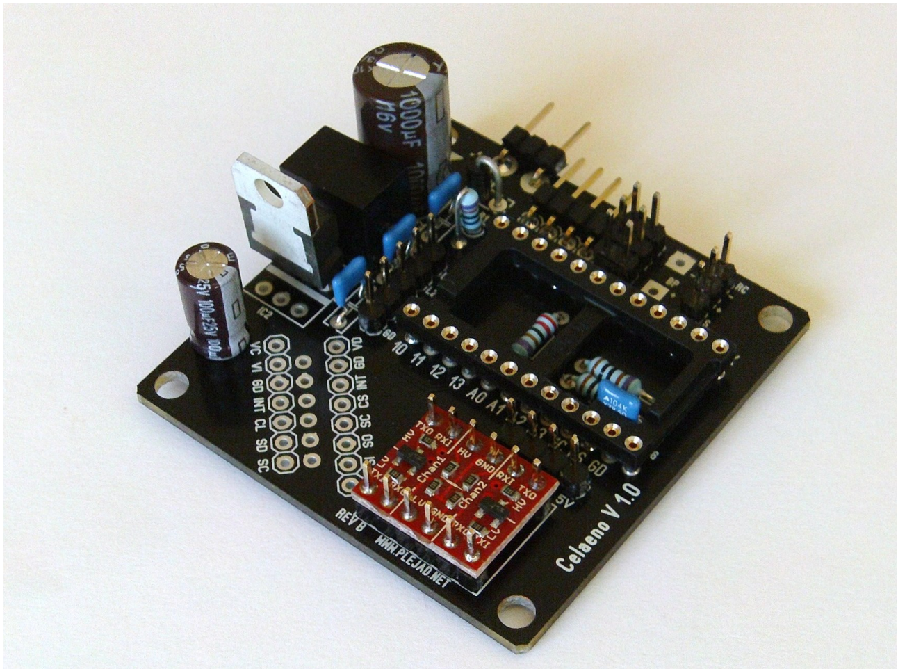
Abbildung 14: Einbau des Pegelwandlers
