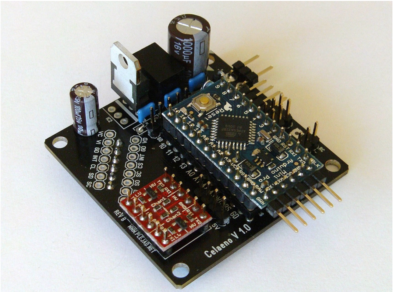
Abbildung 19: Arduino-Einbau
