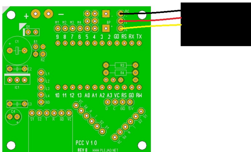
Abbildung 30: Verbindung mit dem Empfänger
