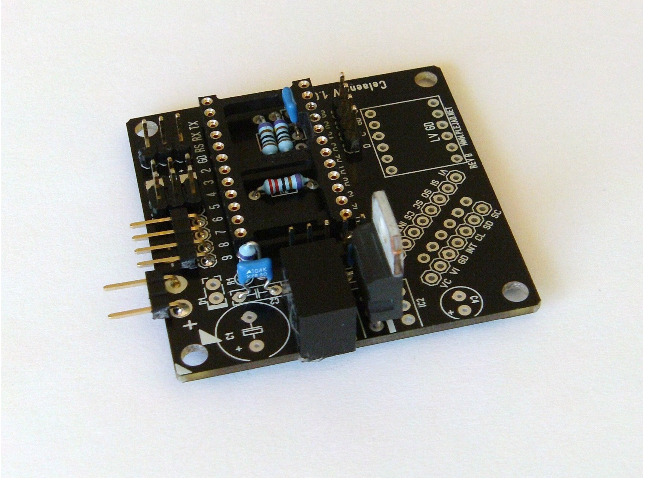
Abbildung 10: Einbau des linearen 3V Spannungswandlers
