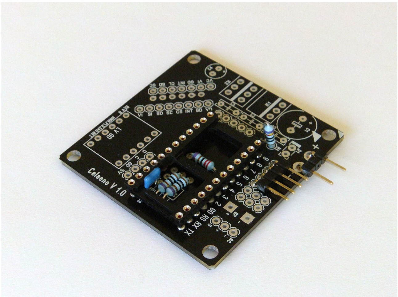
Abbildung 6: Einbau DIL24-Sockel und Stiftleisten
