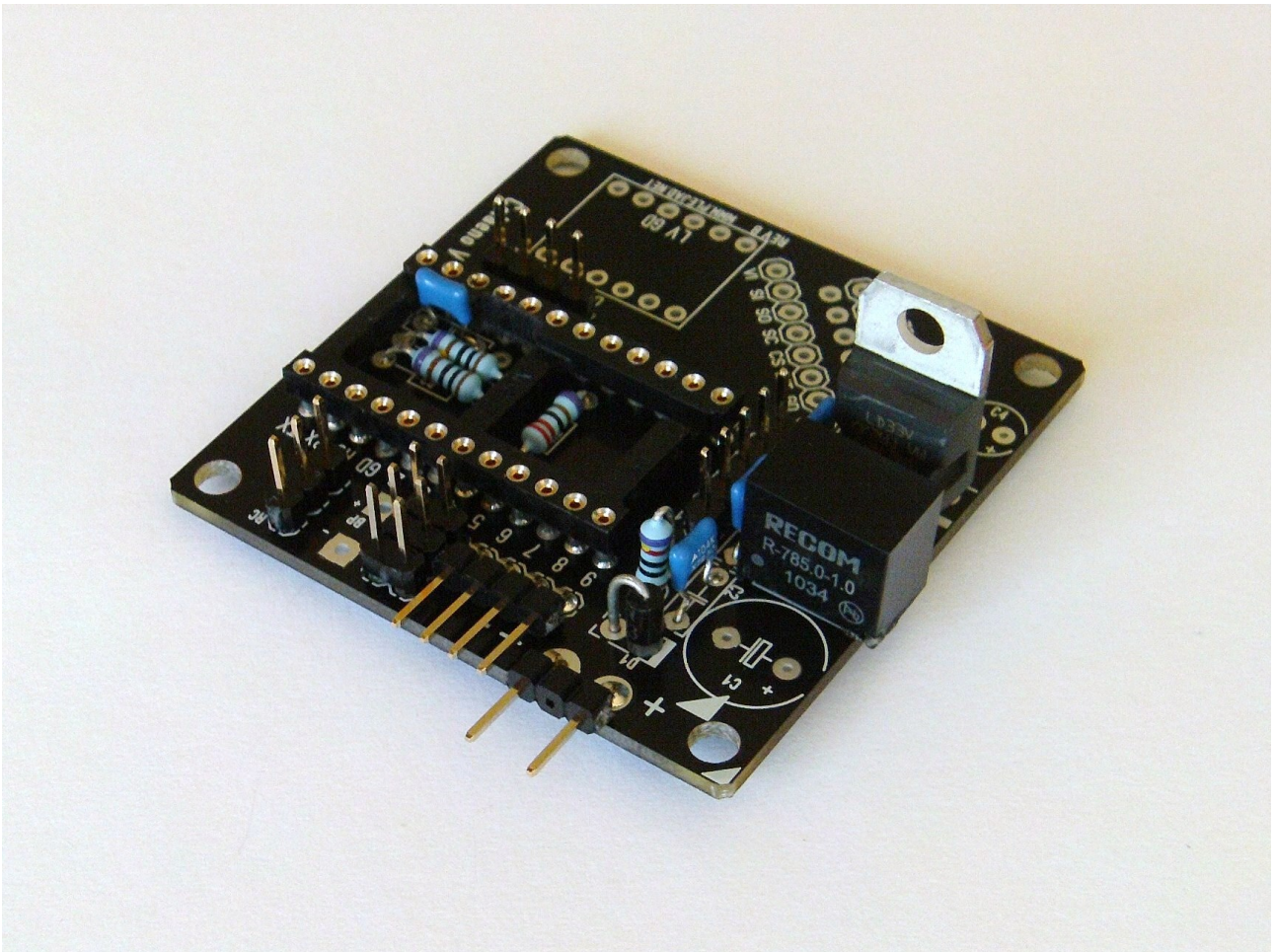
Abbildung 11: Bestückung Diode D1
