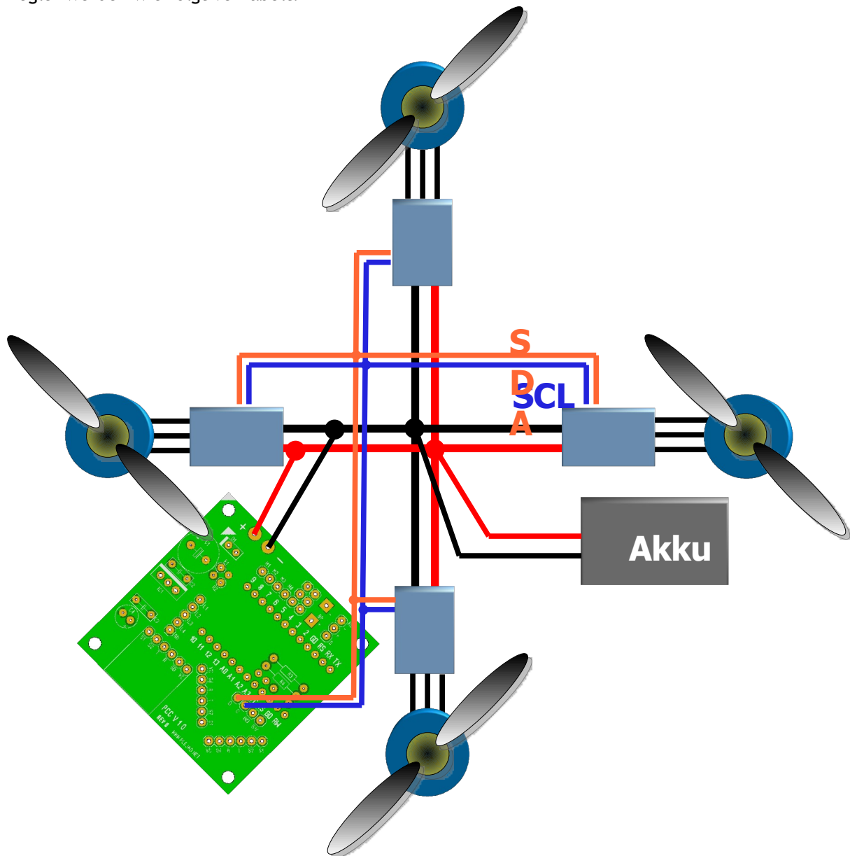
Abbildung 33: I 2 C Regler - Verkabelung
