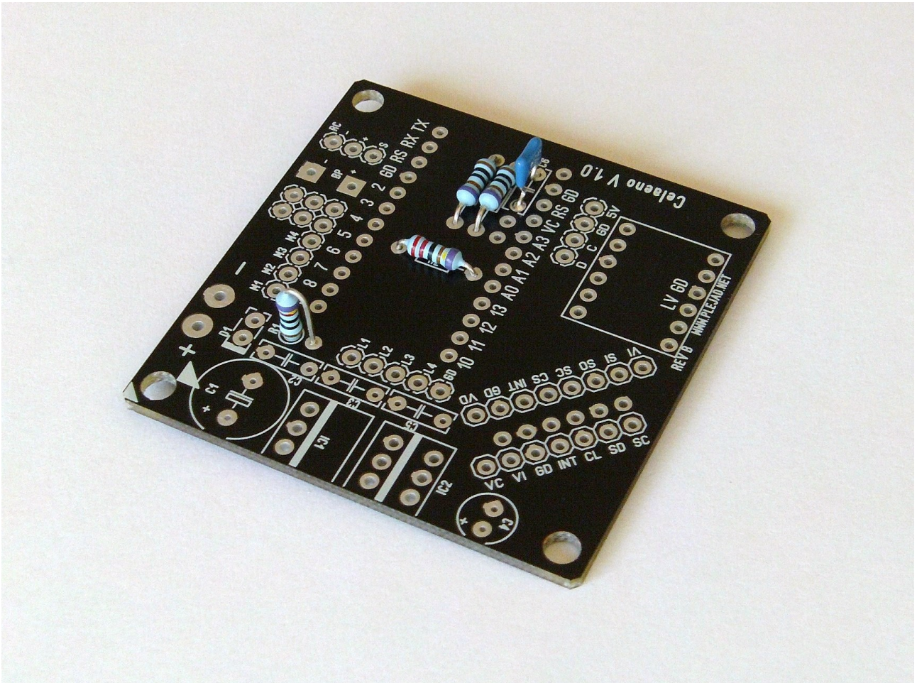
Abbildung 5: Einbau von R1 und R2
