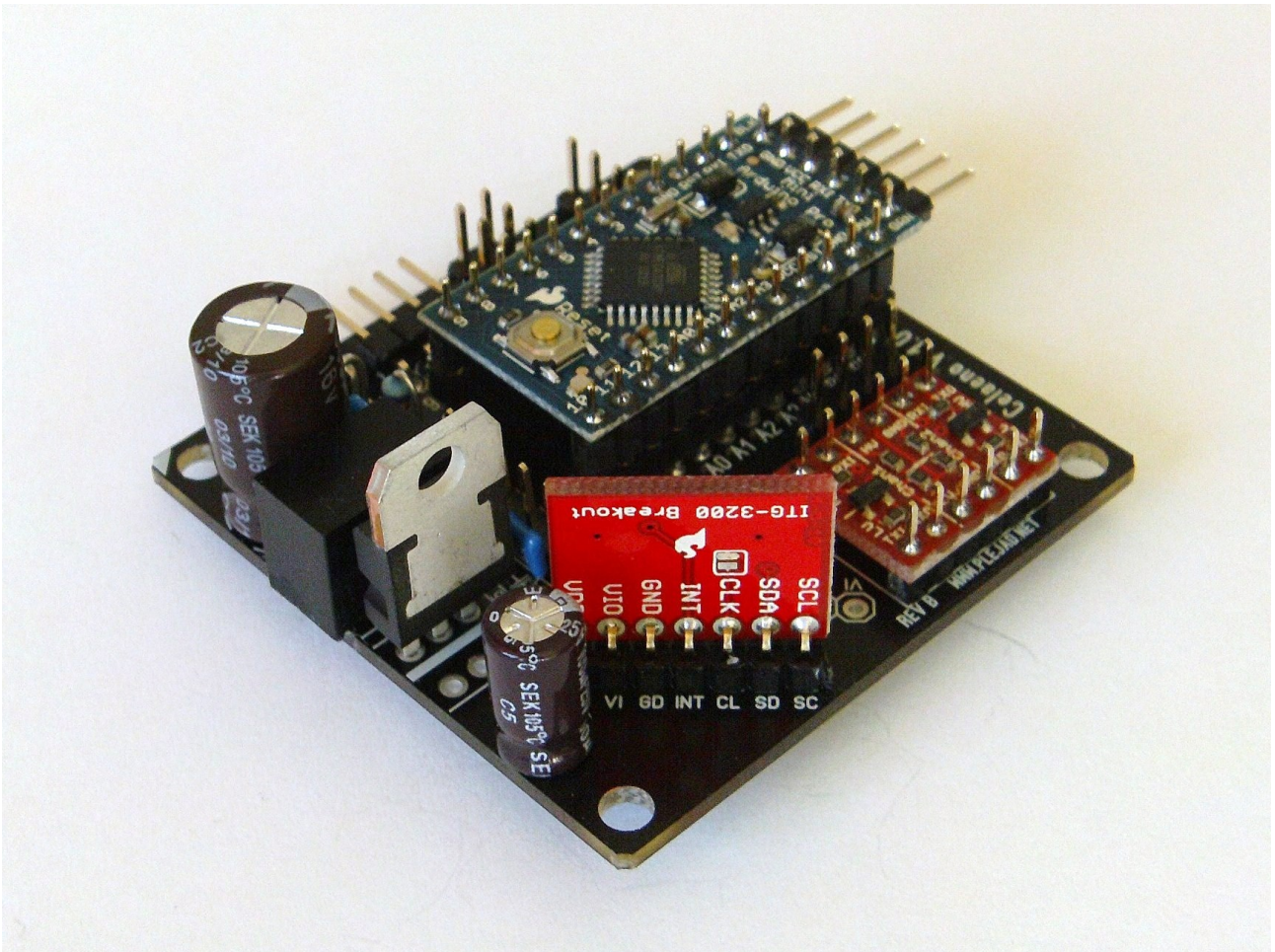
Abbildung 20: Die fertige Platine
