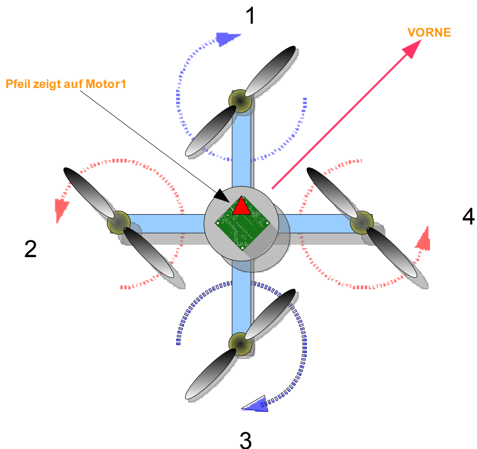
Abbildung 36: Mischer - X Formation
