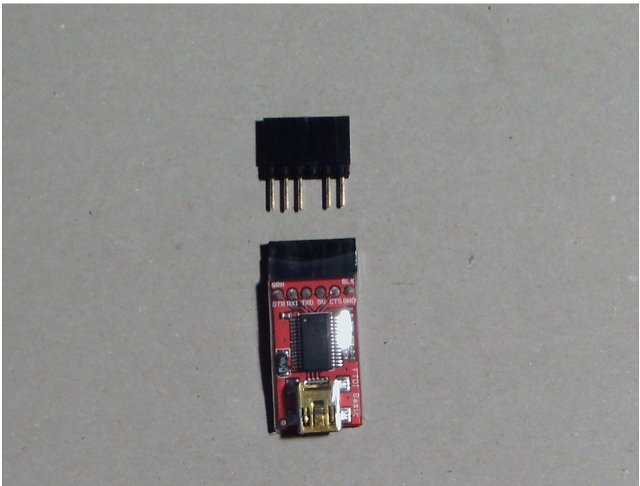
Abbildung 22: Zwischenstecker anfertigen
