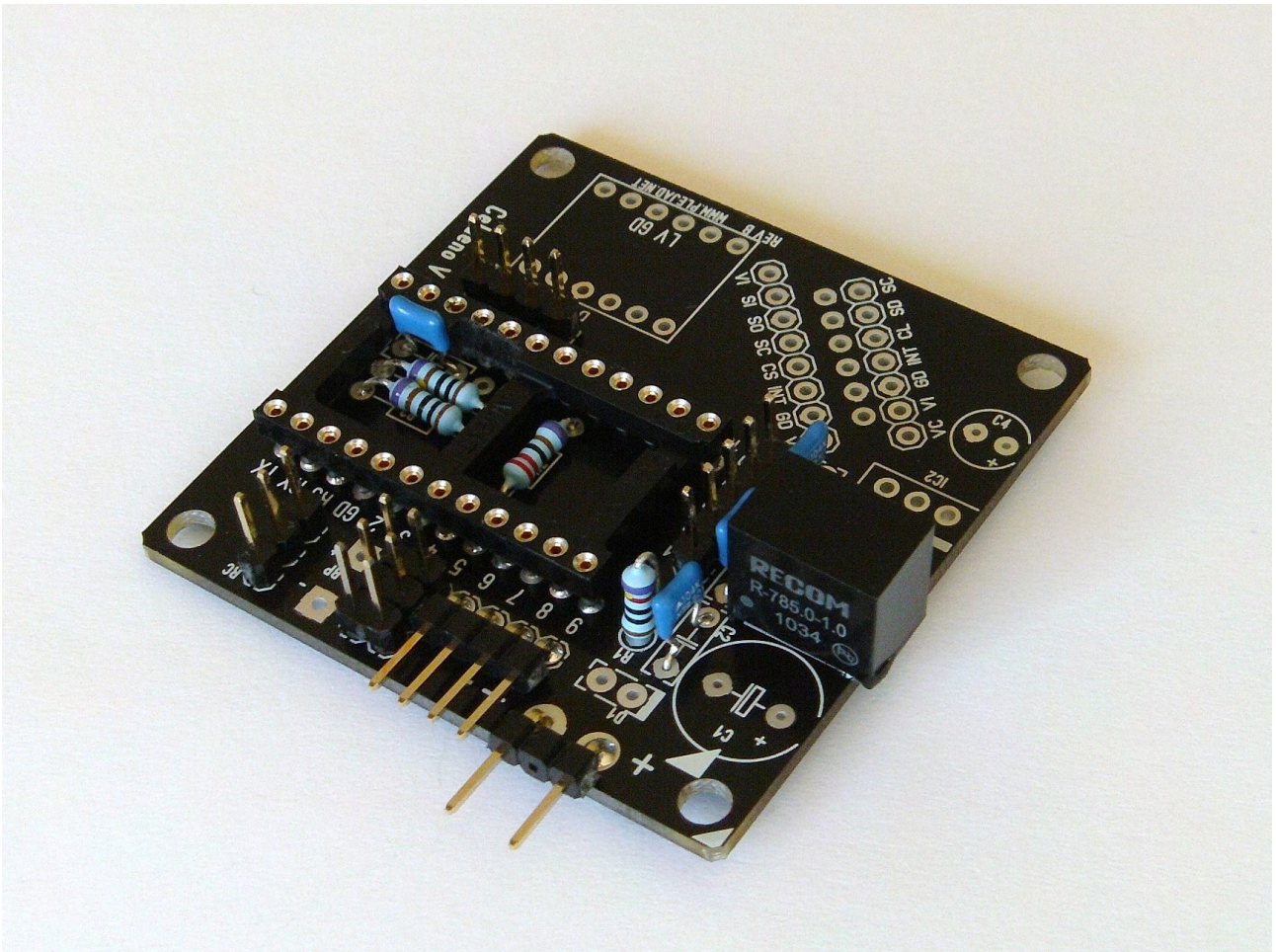
Abbildung 9: Einbau des RECOM Spannungswandlers
