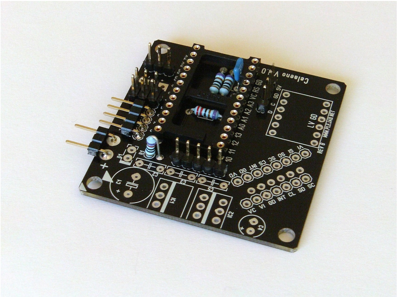
Abbildung 7: Restliche Stiftleisten
