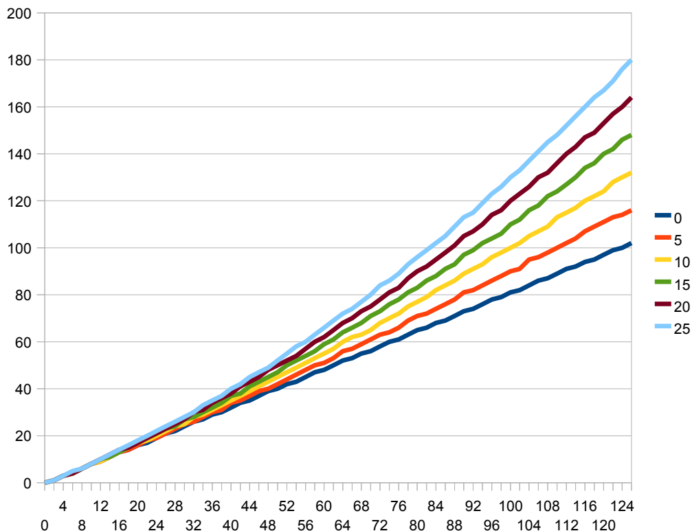
Abbildung 35: E Stick - Exponentialfunktion
