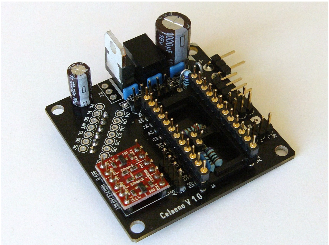
Abbildung 18: Vorbereitung des Arduino-Einbaus
