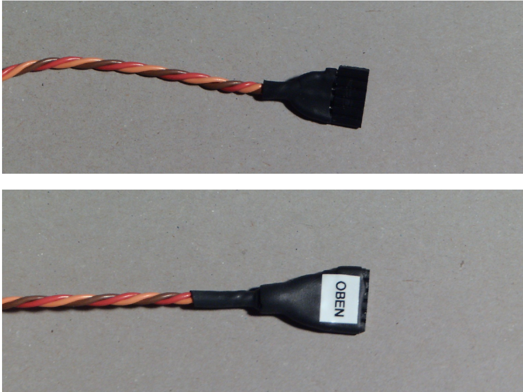
Abbildung 27: Einschrumpfen des Steckers
