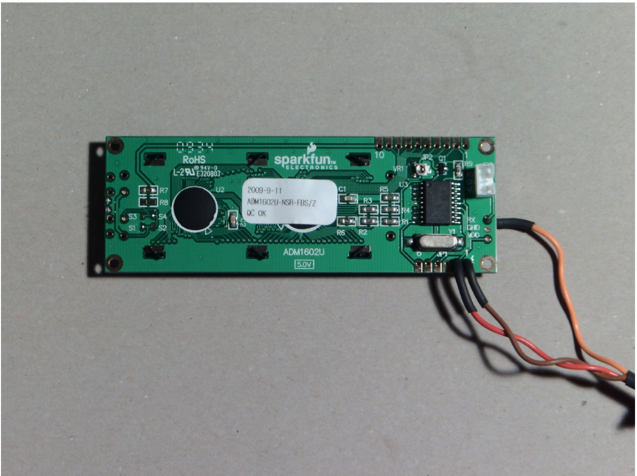
Abbildung 26: Anschluss des LCD Terminals
