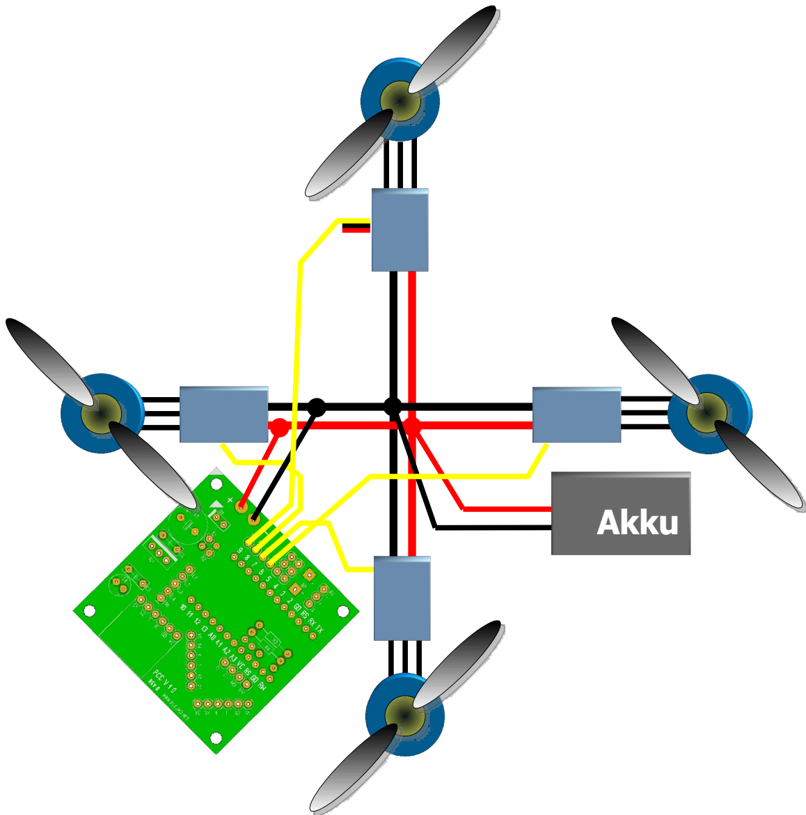
Abbildung : Verkabelung - PWM Standardregler
