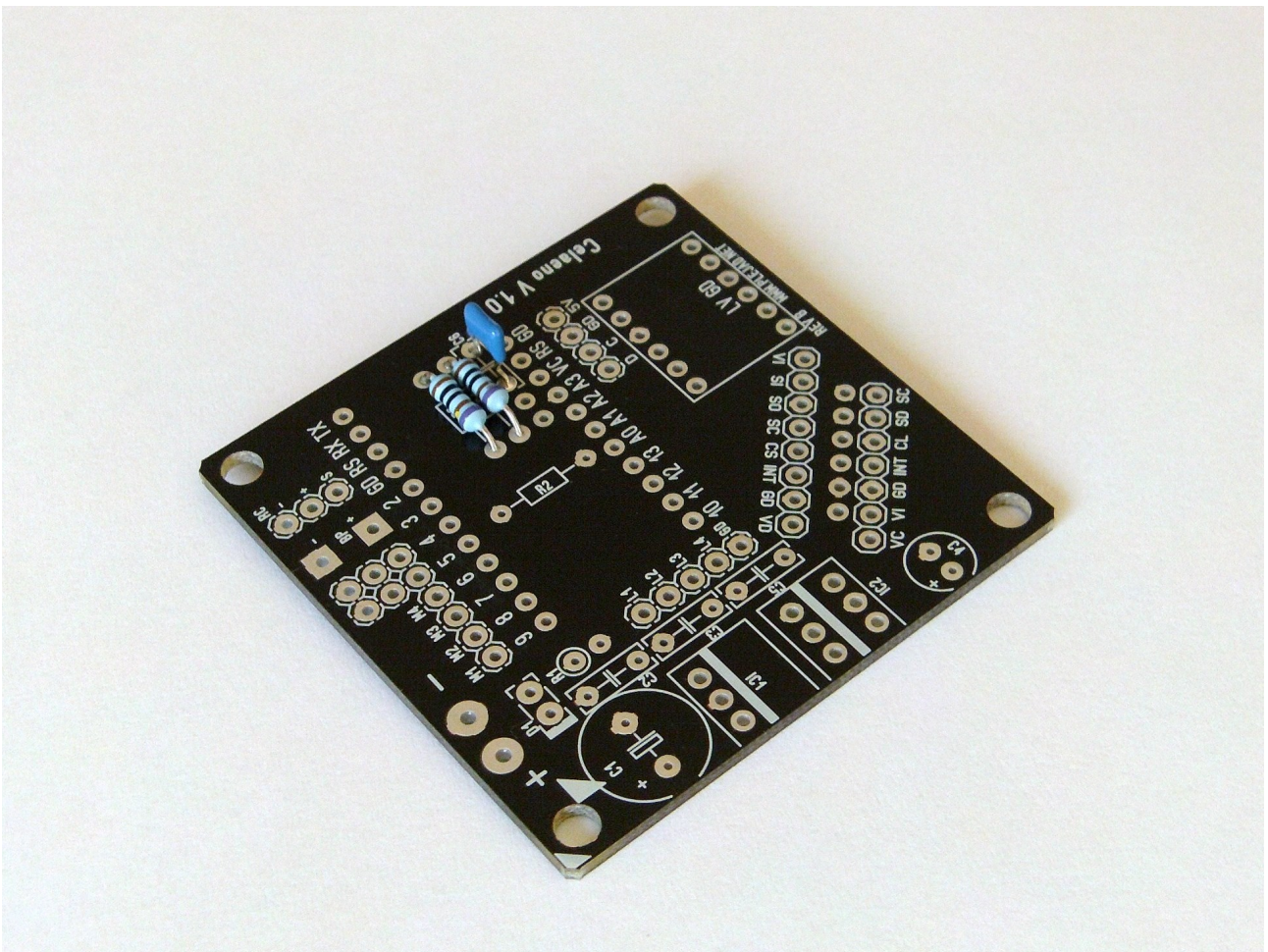
Abbildung 4: Einbau von R3, R4 und C6
