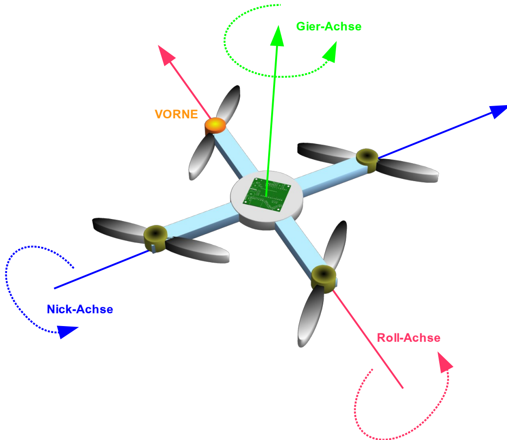
Abbildung 2: Multicopter-Achsen
