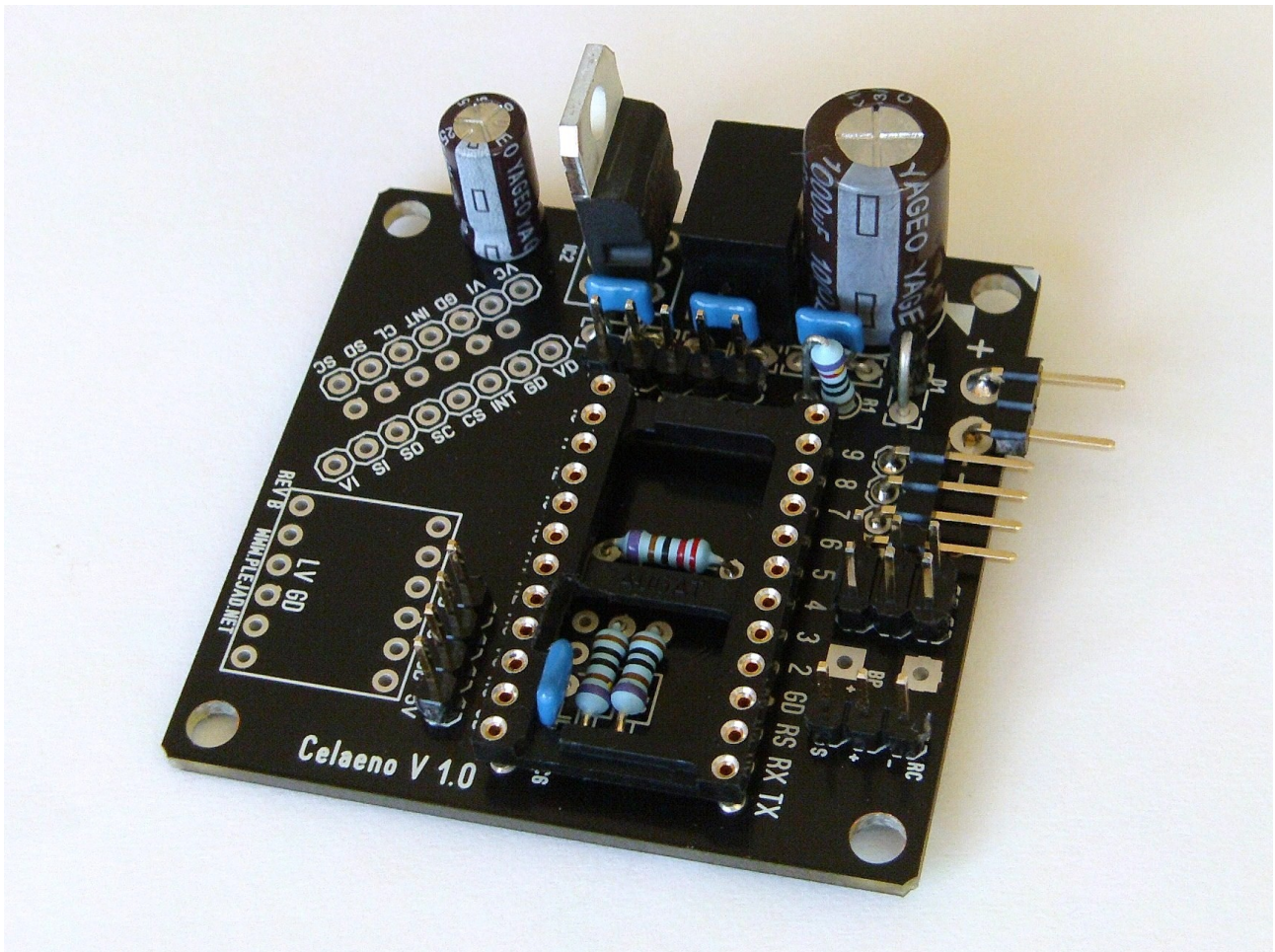
Abbildung 12: Bestückung C1 und C4
