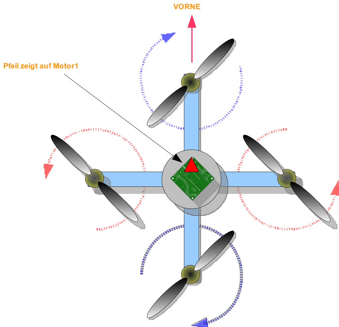
Abbildung 34: Motordrehrichtungen und Platinenausrichtung
